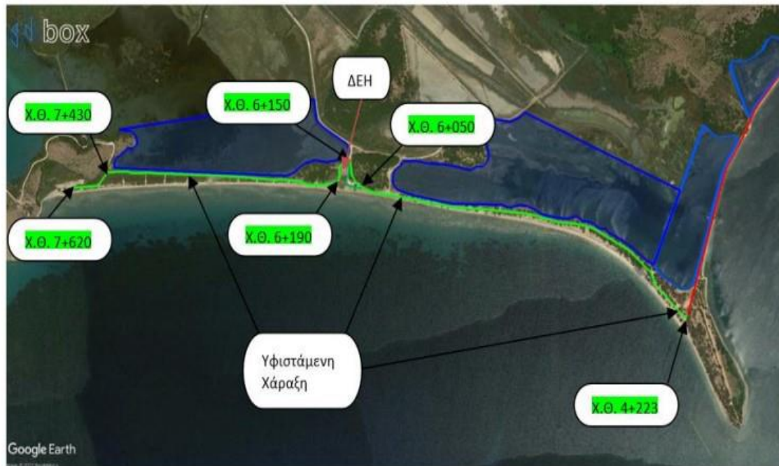
Εικόνα 6-22: Άξονας υφιστάμενης χάραξης - Τμήμα: Δρέπανο - Μακρυγιάλι (Από Χ.Θ. 4+223 έως Χ.Θ. 7+620)
