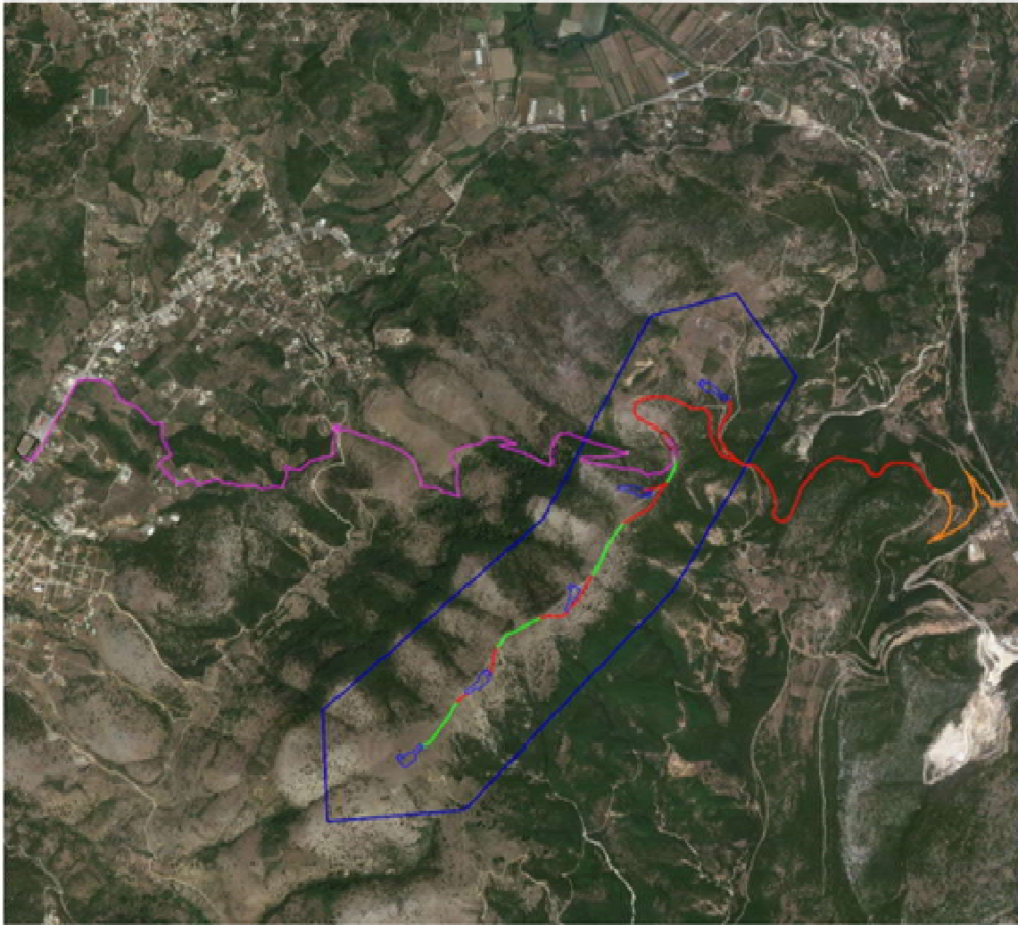
Εικόνα 3.2: Απεικόνιση του πολυγώνου του προτεινόμενου αιολικού πάρκου, των οδών πρόσβασης και με ματζέντα άδευση του δικτύου διασύνδεσης (πηγή: Google earth, επεξεργασία)
