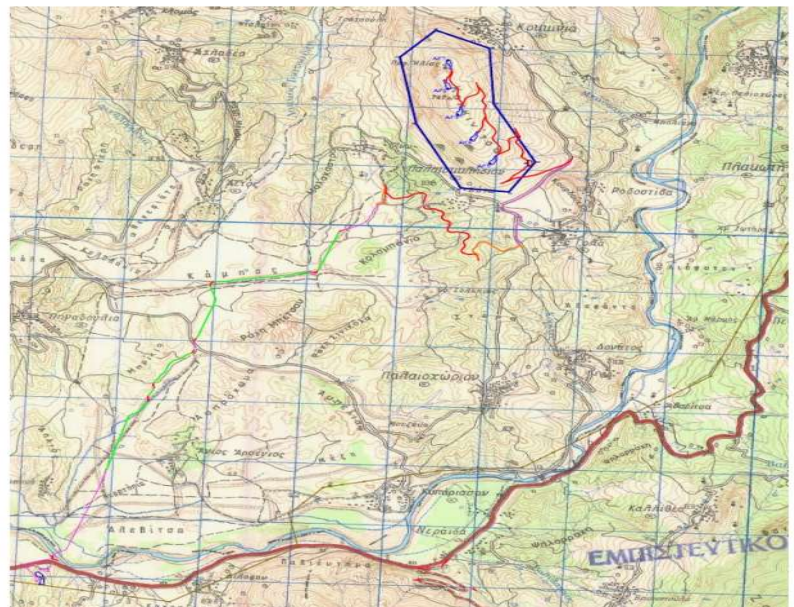
Εικόνα 2: Απόσπασμα Χάρτη προανατολισμού με αποτύπωση του αιολικού πάρκου της οδοποιίας πρόσβασης (κόκκινη οδευση) και της διασύνδεσης (ματζέντα οδευση, (υπόβαθρο: ΓΥΣ, επεξεργασία)
