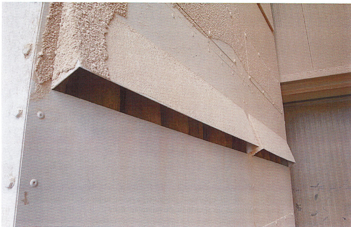
Εικ.2 Σύστημα αναρρόφησης σκόνης στο χώρο παραλαβής πρώτων υλών
